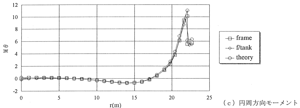
図-5 底版の計算結果
