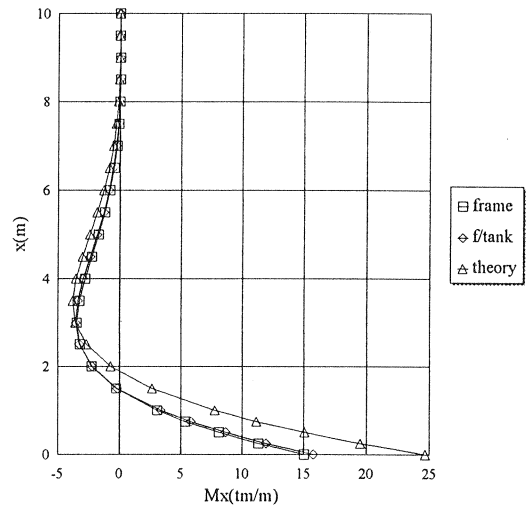
(c) 鉛直方向曲げモーメント
