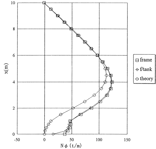
(b) 円周方向軸力
