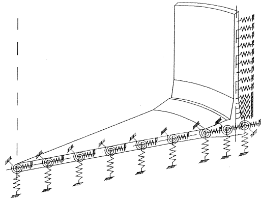
図-1 構造のモデル化
