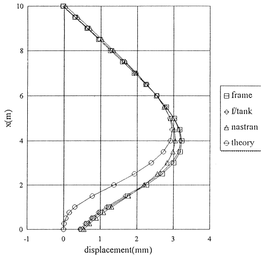
(a) 半径方向変位
