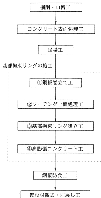
図-8 NP-3, 4橋脚の施工フロー
