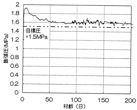
図-3 実物大模型の温度と膨張圧の経時変化
