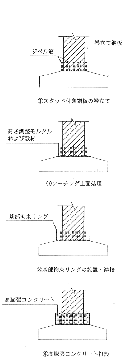
図-9 基部拘束リングの施工順序
