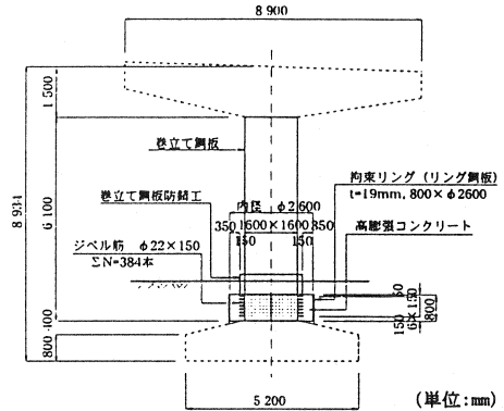
図-6 NP-3.4 橋脚構造図
