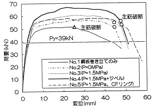
図-5 荷重変位包絡線
