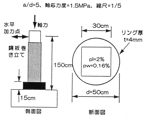
図-4 縮小模型の概要
