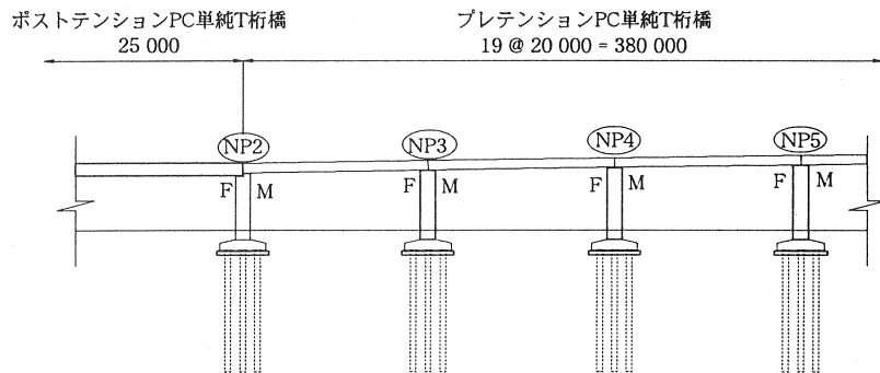
図-7 洲崎高架橋側面図
