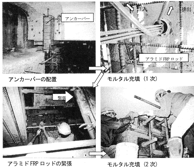
写真-7 変位制限構造の施工
