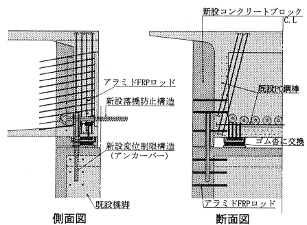
図-1 主橋梁部補強詳細図 (P0, P6)
