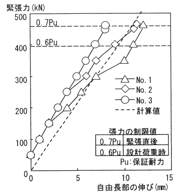
図-6 現場引張り試験結果の例
