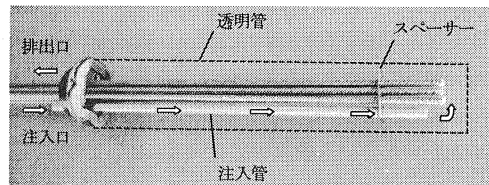
写真-4 アラミドFRPロッドの配置
