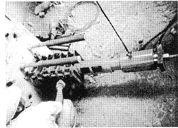
写真-6 現場引張試験状況
