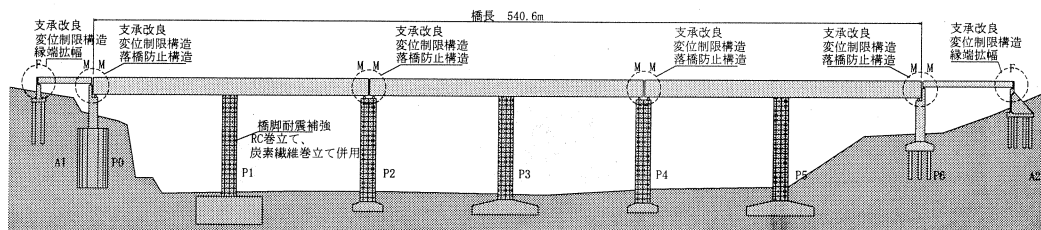
図-2 補強概要
