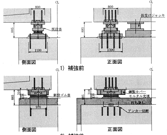
図-3 新旧支承構造図
