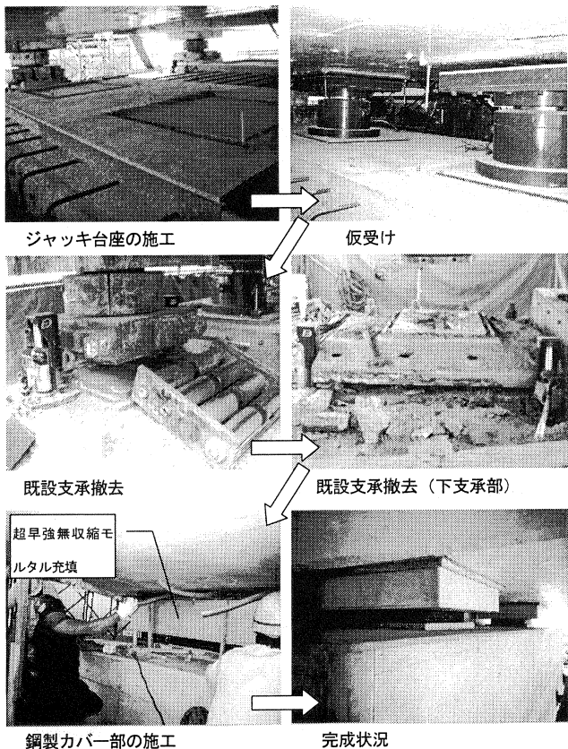
写真-2 支承交換状況
