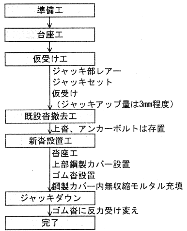
図-4 支承交換手順
