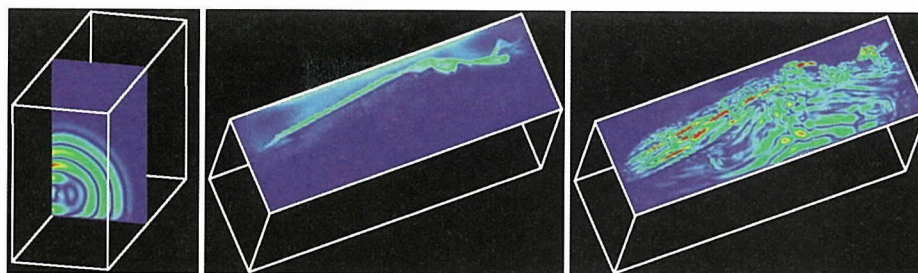
図-3 大規模FEM地質モデル(1000万自由度)の波動伝播解析(速度分布センター)
