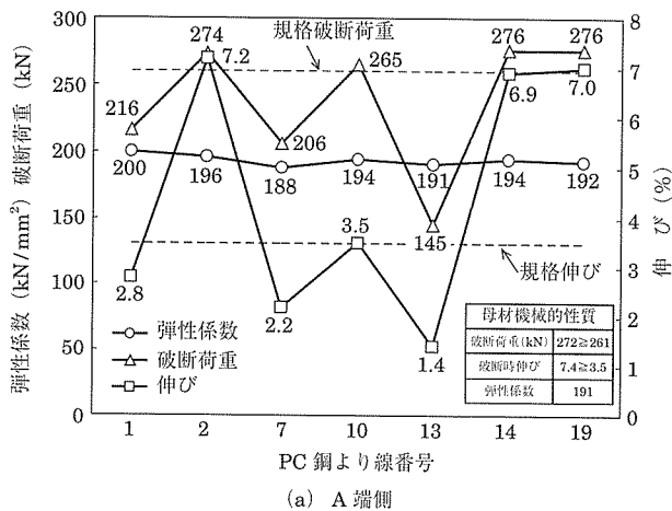
図 - 12 破断荷重と伸びの関係 (CASE - 4)
