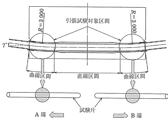
図 - 5 引張試験対象区間
