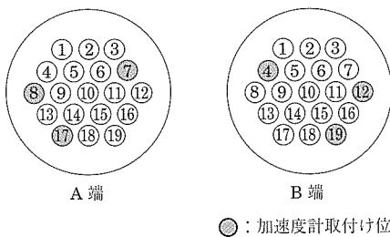
図 - 4 加速度計を取付けた PC 鋼より線番号
