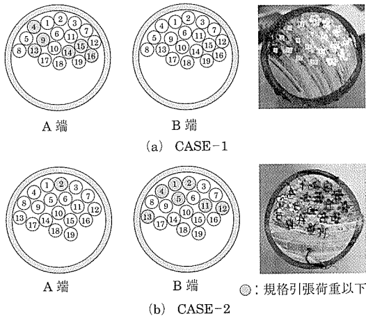
図 - 6 ケーブル断面 (中央部)
