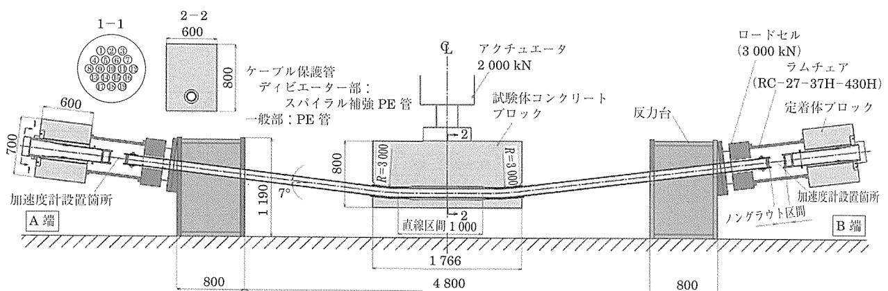
図-3 試験装置全景
