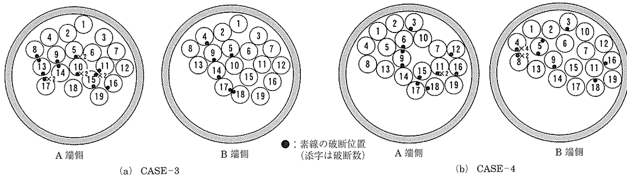
図 - 11 試験体側面に対する素線の破断位置
