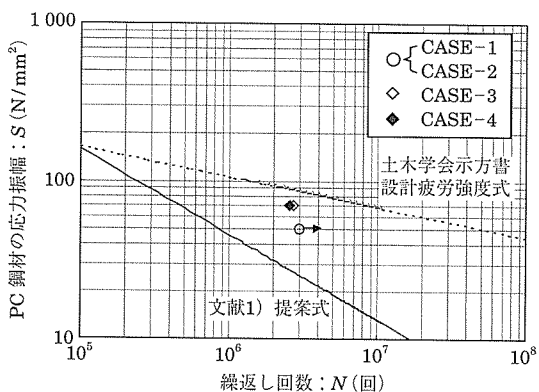
図-7 PC鋼より線の疲労強度式 (初破断時)
