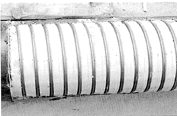
写真 - 6 スパイラル補強 PE 管内のグラウト充填状況
