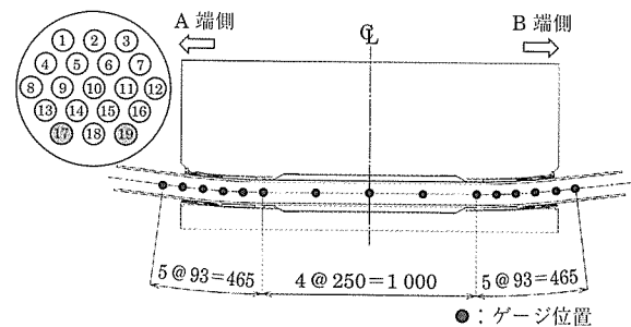
図 - 13 ゲージ貼付け位置
