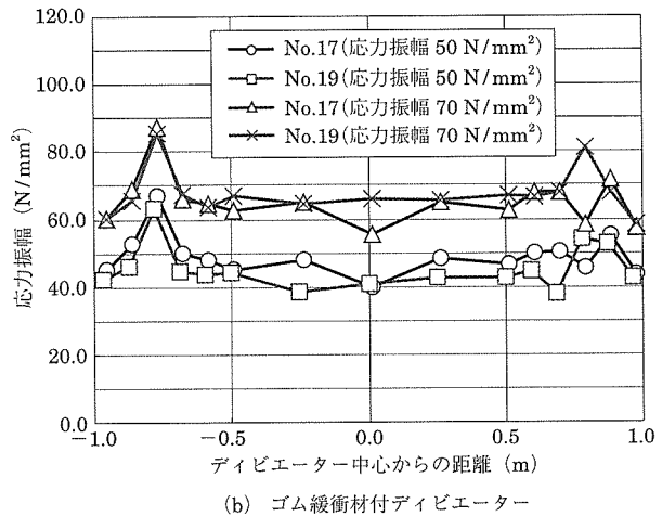
図 - 14 ディバイエーター内 PC 鋼より線の応力振幅測定結果
