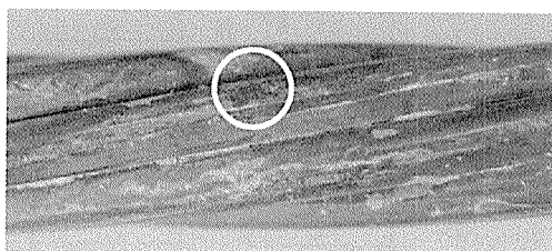
(b) フレッシングコロージョン (赤錆)
