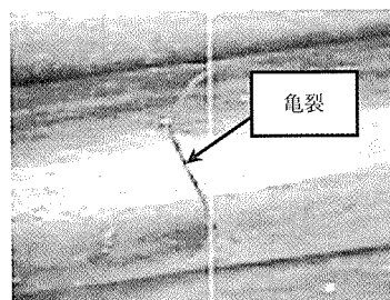
写真 - 5 引張試験後に確認された素線の亀裂 (※中央の白線は撮影機の走査線)
