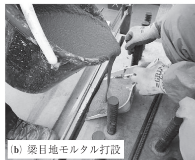
写真 - 7 PCaRC 柱・PCaPC 梁目地打設および PC 緊張状況
