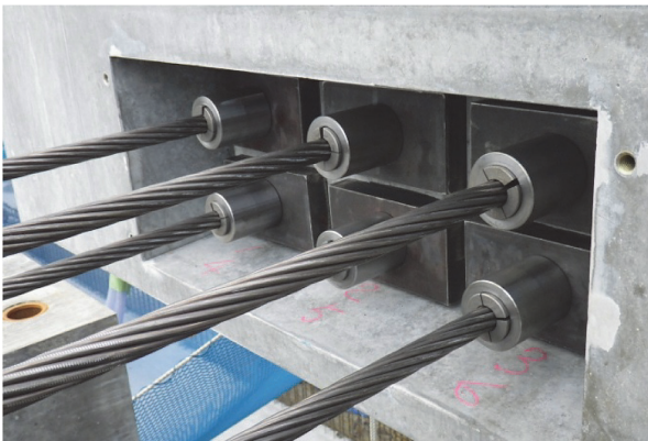
写真 - 2 シングルストランド定着具納まり状況
