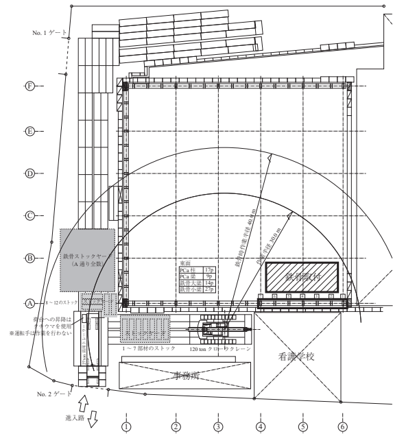
図 - 9 架設計画図（A 通り側の場合）
