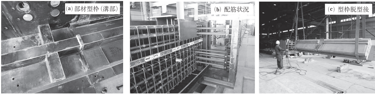
写真 - 3 PCa 部材の製作状況
