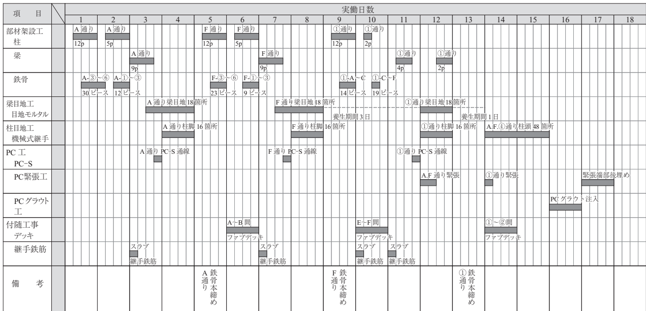
図 - 11 1層分のサイクル工程
