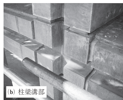
写真 - 8 PCa 部材仕上げ状況
