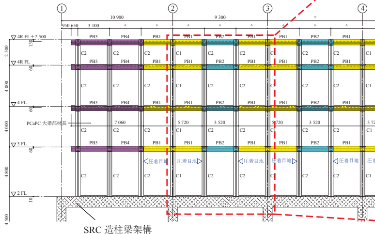
図 - 6 PCa 架構の部材分割計画概要
