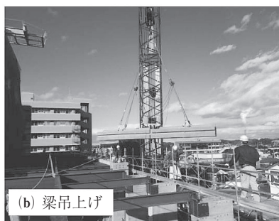
写真 - 6 PCaPC 梁の架設状況
