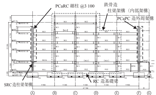
図 - 5 3 通り軸組図
