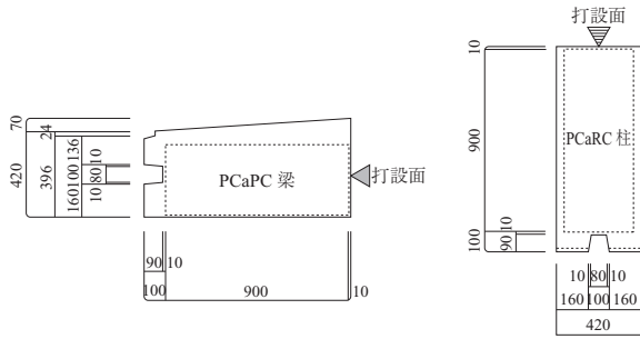
図 - 7 PCa 部材形状図
