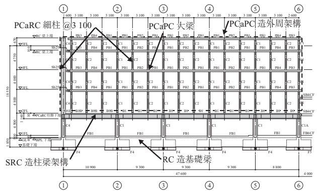
図 - 4 A 通り軸組図
