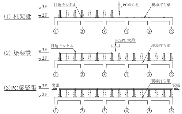
図 - 10 架設手順図
