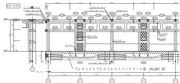
図 - 11 陸立ち架構の軸組図
