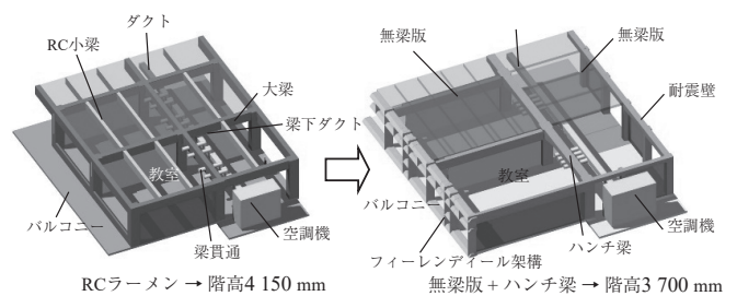
図 - 3 構造と設備ルート
