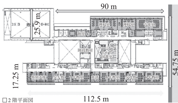
図 - 1 平面図
