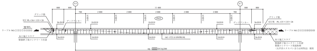
図 - 12 PRCスラブの配線配筋図
