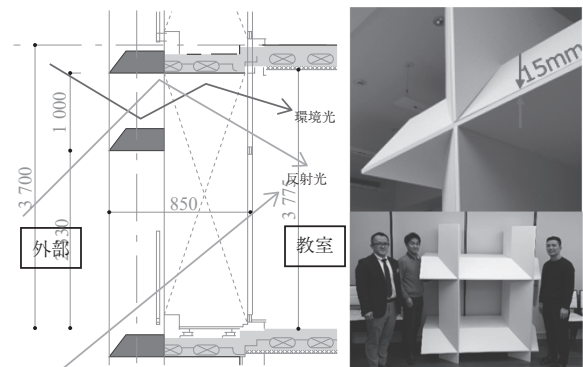
図 - 4 フィーレンディール形状スタディ
