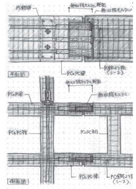
図 - 19 目地モルタル用型枠要領 図 - 20 PC 接続イメージ
