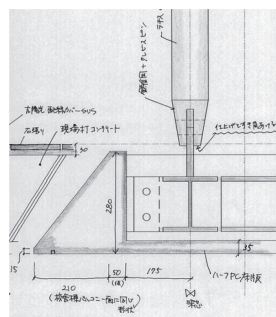
図 - 6 連絡橋ディテール
