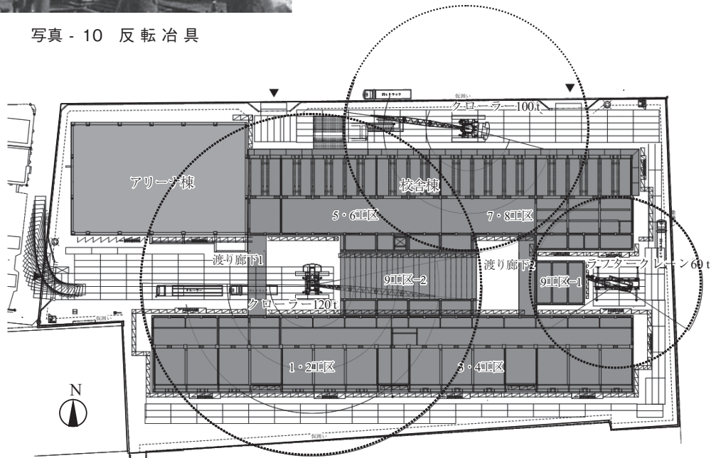
図 - 15 仮設計画図
