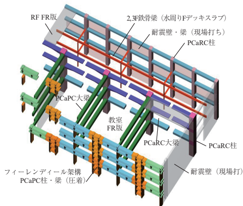
図 - 9 PCa 部材の概要図 (教室)
