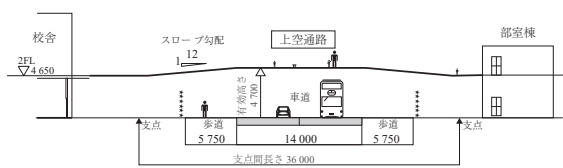
図 - 5 連絡橋の設計条件
