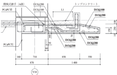
図 - 13 底PCa版断面図
