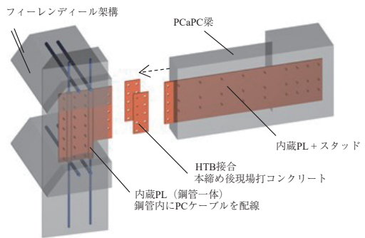
図 - 10 PCaPC 架構の接合部納まり
