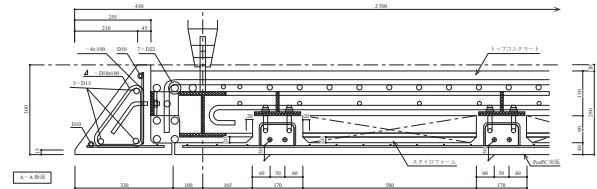
図 - 14 連絡橋のハーフPCa床版
