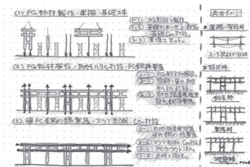
図 - 16 初期段階の建て方イメージ
